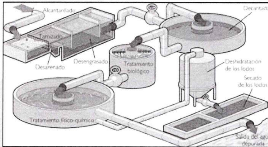
Gráfico 10: Procesos del tratamiento de aguas servidas Fuente: Synergy, Agua y Energía
