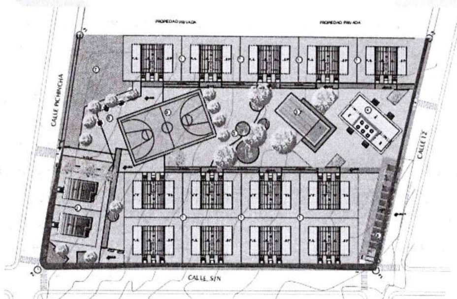
Gráfico 2: Implantación del proyecto San Sebastián, cantón Colta, Chimborazo
