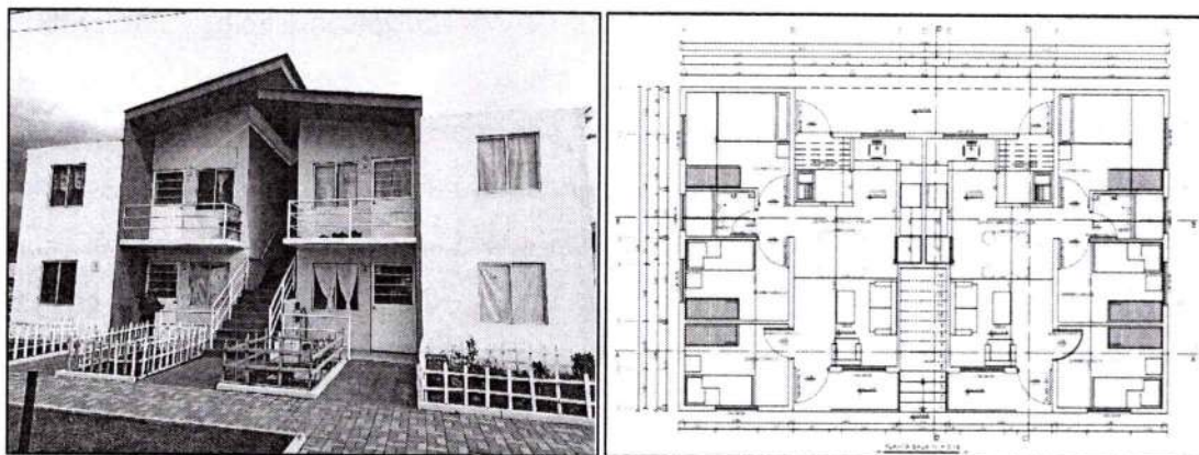
Gráfico 3: Edificio multifamiliar 4D del proyecto San Sebastián, cantón Colta, Chimborazo
