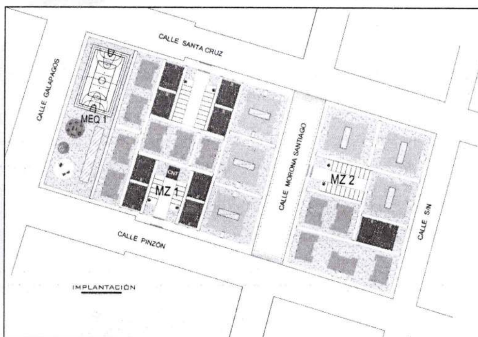
Gráfico 5: Implantación de las soluciones habitacionales construidas en la parroquia El Triunfo, cantón La Maná, Cotopaxi
