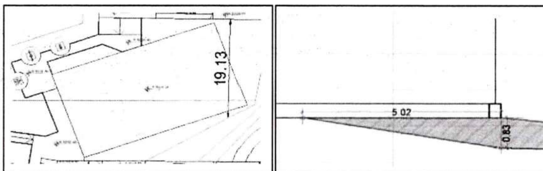
Gráfico 7: Perfil de relleno compactado en el área de cancha
