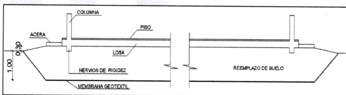
Gráfico 11: Geometría del relleno con sub base clase 3
